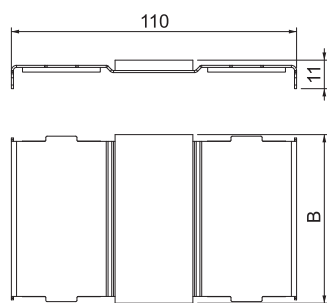
Abmessungen
