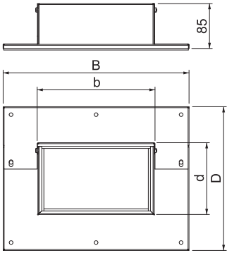
Abmessungen
