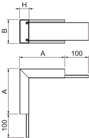
Abmessungen
