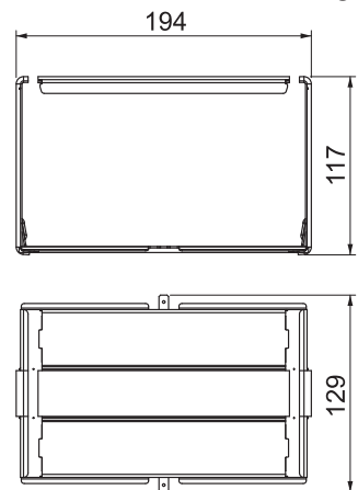
Abmessungen
