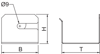
Abmessungen
