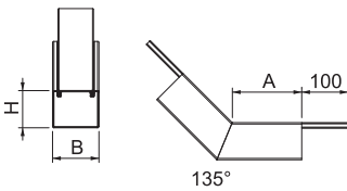
Abmessungen
