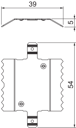
Abmessungen
