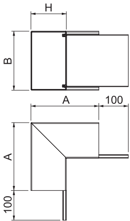
Abmessungen
