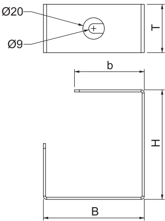
Abmessungen
