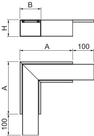
Abmessungen
