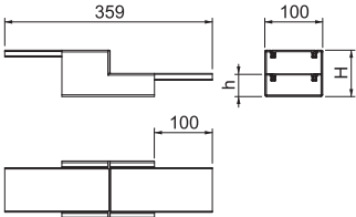
Abmessungen
