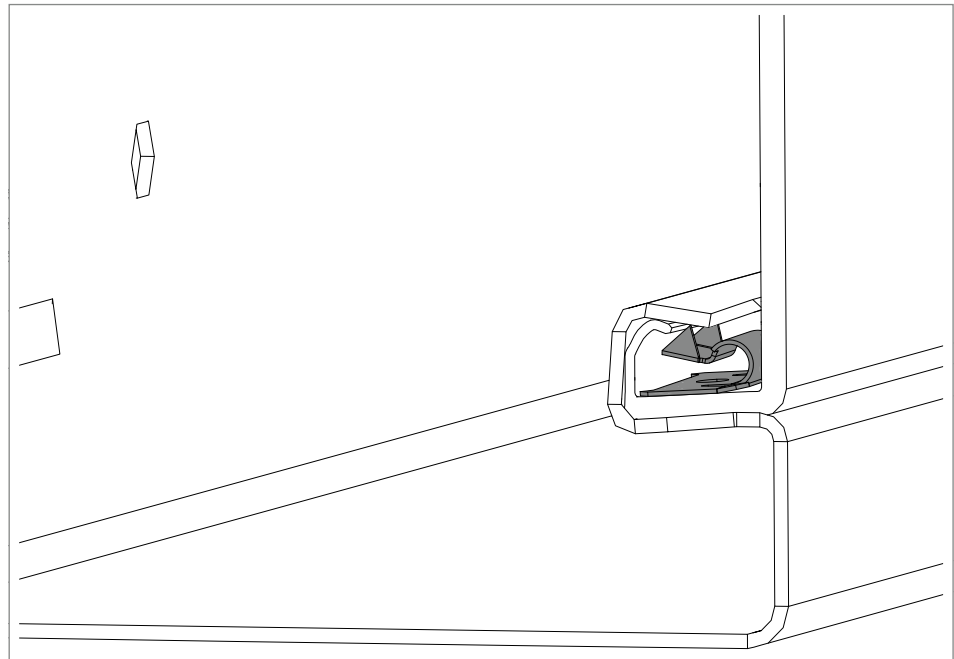
Abb. 3: Rastklammern montieren
