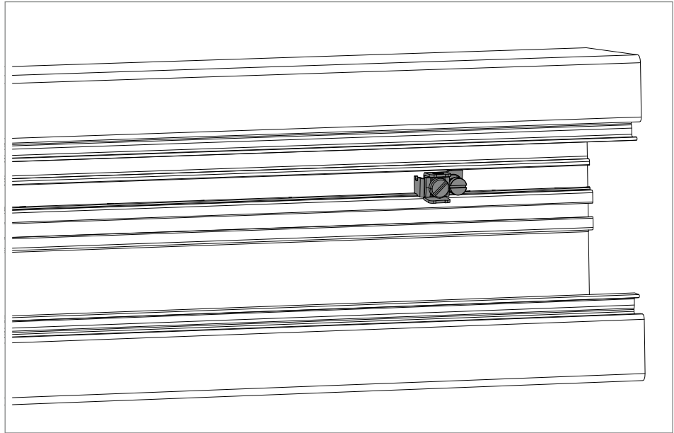
Abb. 2: Schutzleiteranschlusswinkel montieren - Geräteeinbaukanal Aluminium
