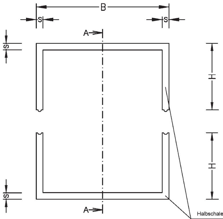
Vorderansicht:
