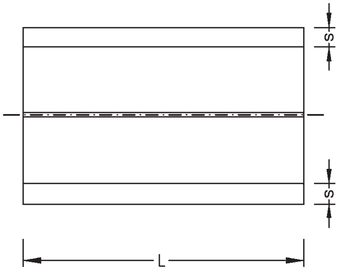
Seitenansicht:
