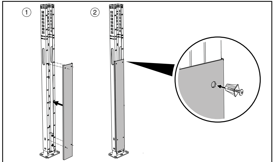
Abb. 42: Deckel montieren
