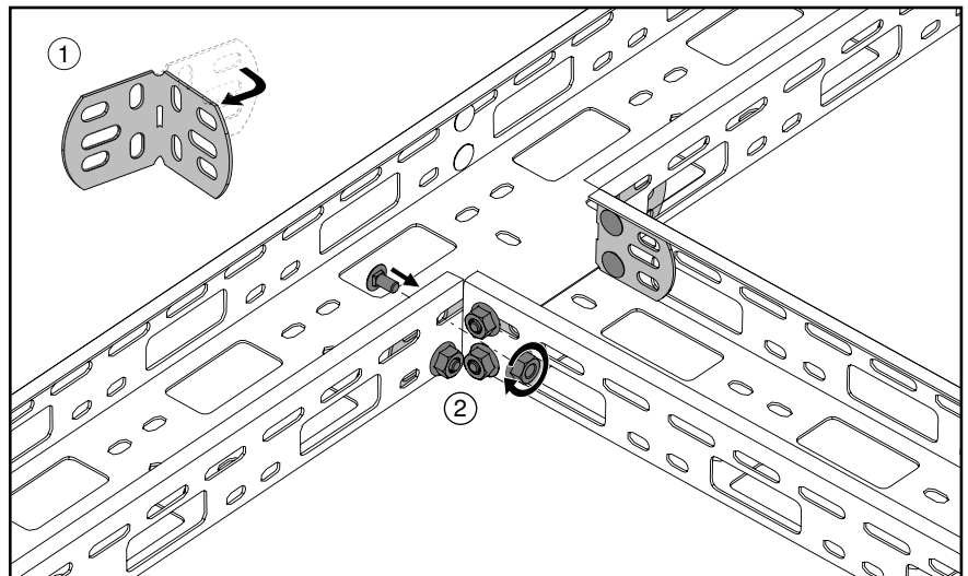
Abb. 29: T-Abzweig montieren
