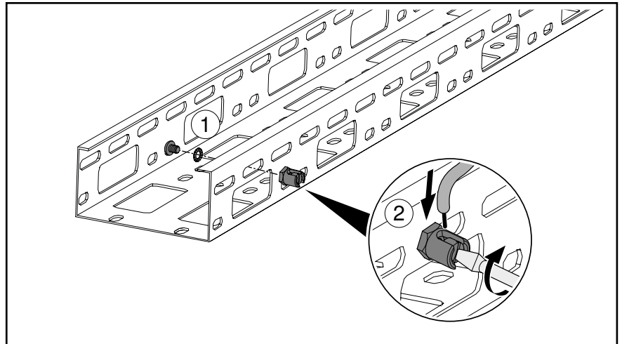
Abb. 44: Erdungsklemme montieren
