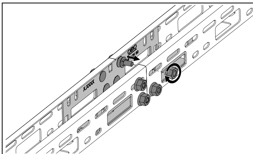
Abb. 16: Längsverbinder montieren
