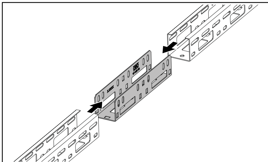
Abb. 15: Längsverbinder positionieren
