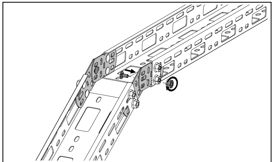
Abb. 22: Gelenkverbindung montieren
