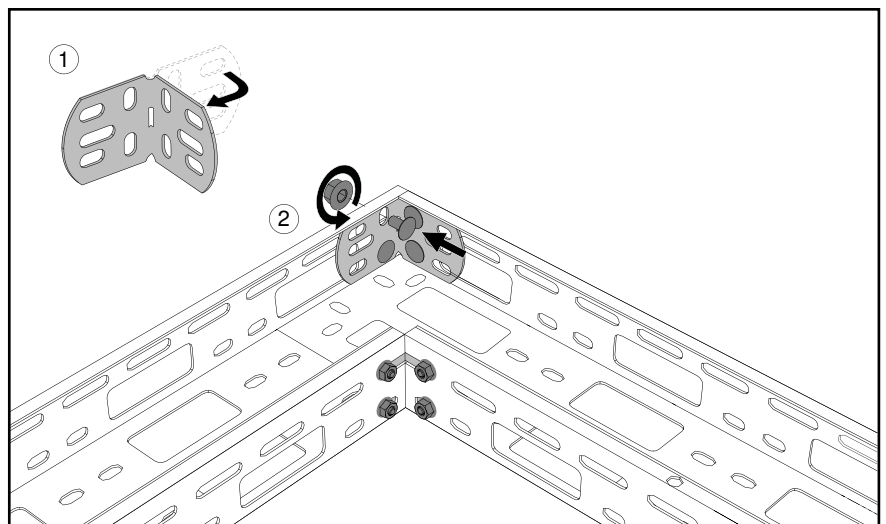
Abb. 18: 90°-Ecke montieren.
