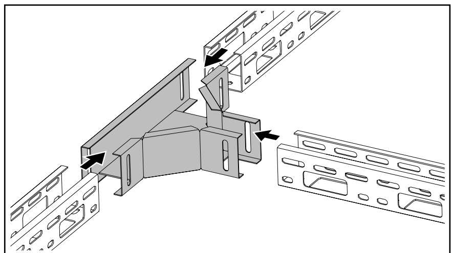
Abb. 30: AZ-Kleinkanäle positionieren
