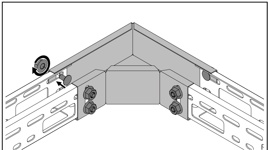
Abb. 20: 90°-Ecke montieren
