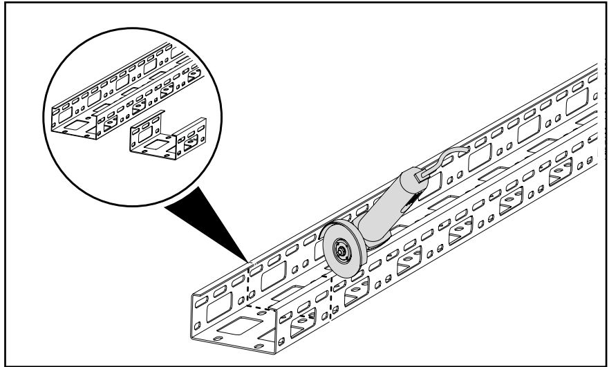
Abb. 23: AZ-Kleinkanal zuschneiden
