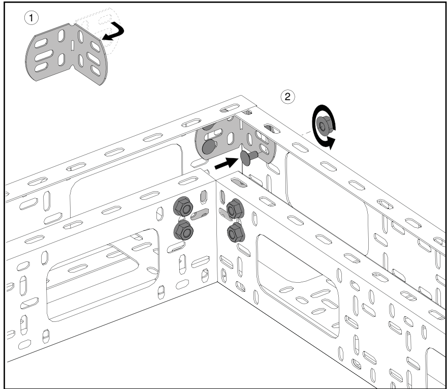
Abb. 9: 90°-Ecke erstellen
