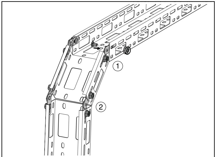
Abb. 24: Scharnierverbinder montieren
