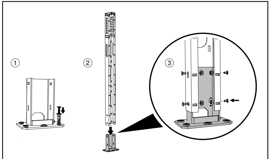
Abb. 39: Säulenfuß montieren
