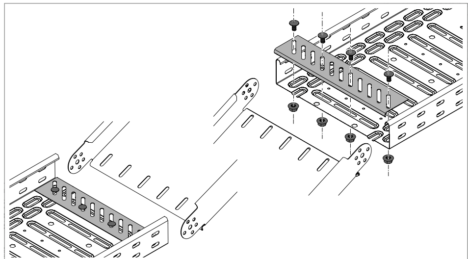
Abb. 70: Bodenendblech montieren
