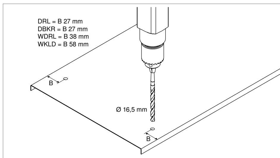
Abb. 86: Deckel vorbohren
