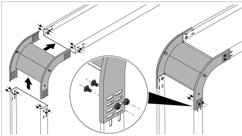
Abb. 67: Fallenden Vertikalbogen montieren
