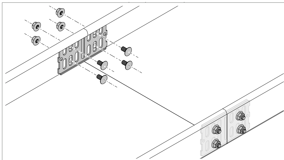
Abb. 26: Längsverbinder RLVK anschrauben
