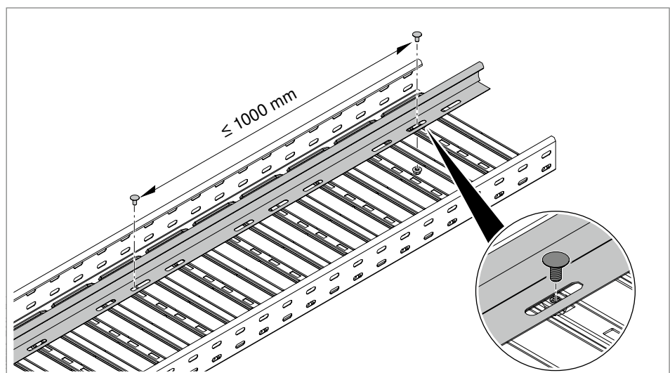
Abb. 78: Trennsteg anschrauben
