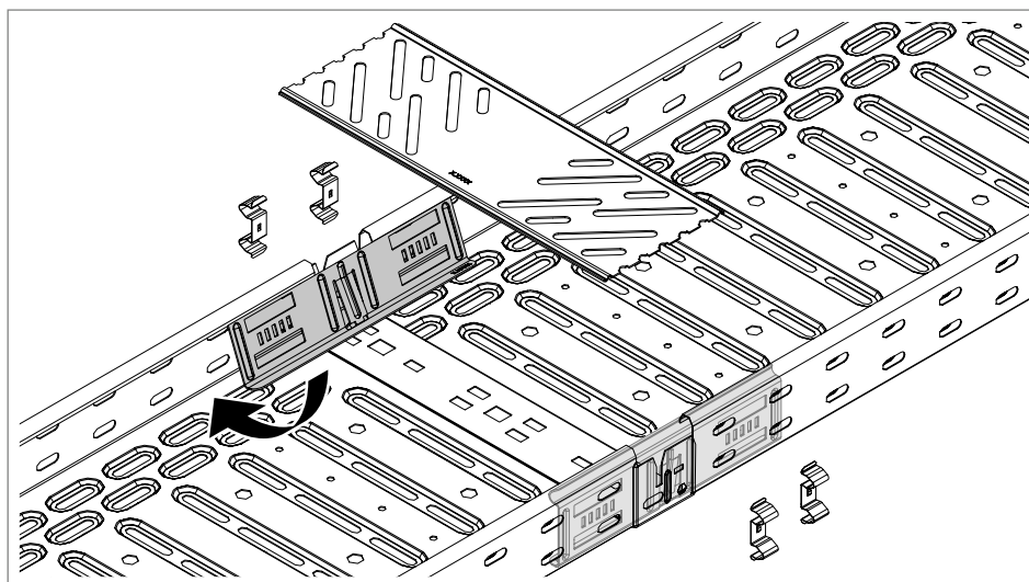
Abb. 22: Längsverbinder KTSMV einsetzen
