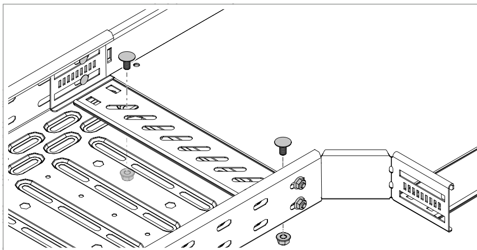
Abb. 54: Stoßstellenleiste anschrauben
