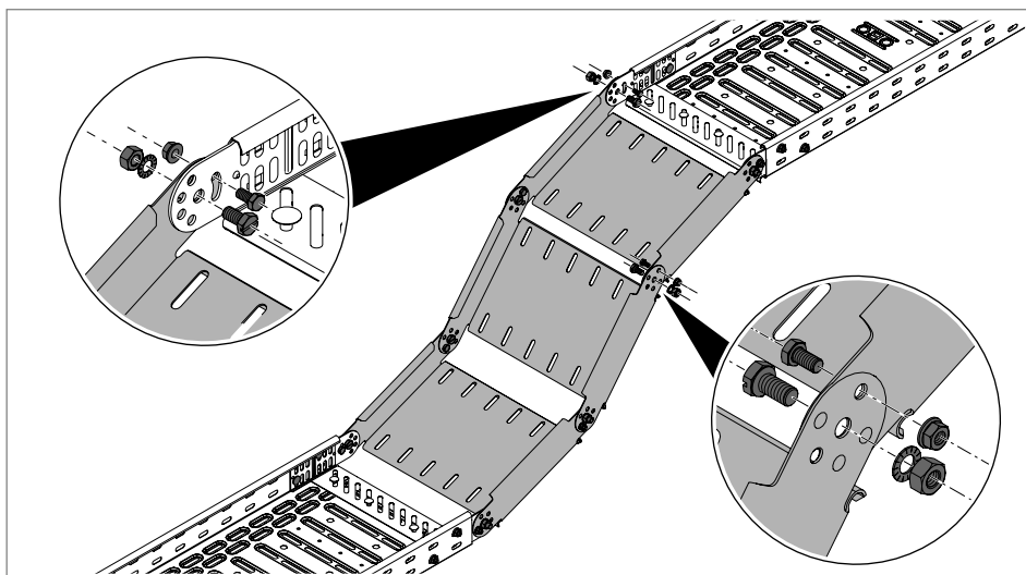
Abb. 72: Gelenkbodenelemente montieren
