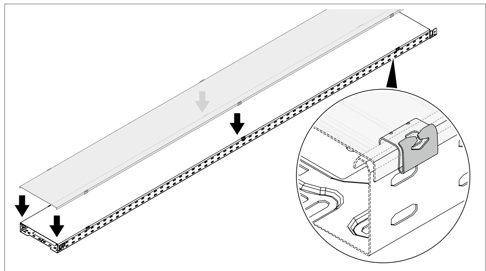
Abb. 85: Deckel aufrasten
