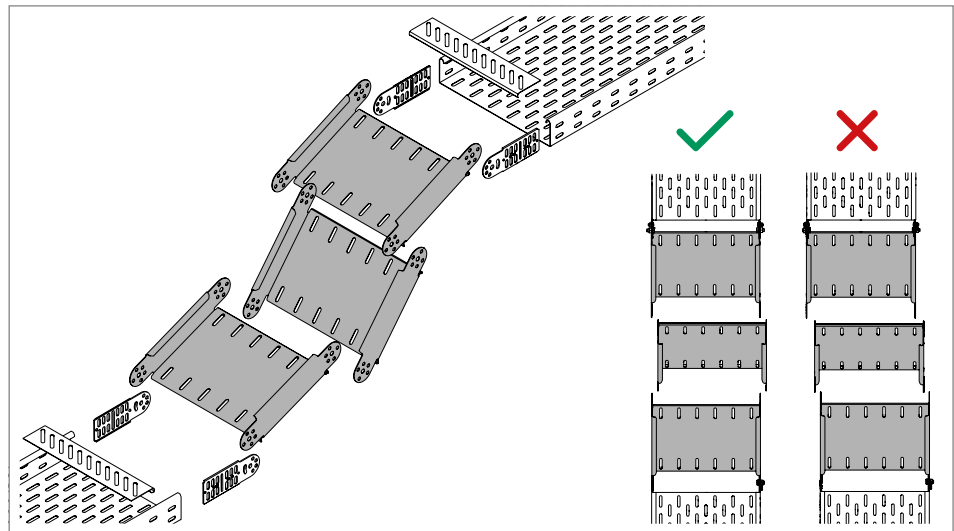
Abb. 69: Gelenkbogenelement mit halben Gelenkverbinder und Bodenendblech
