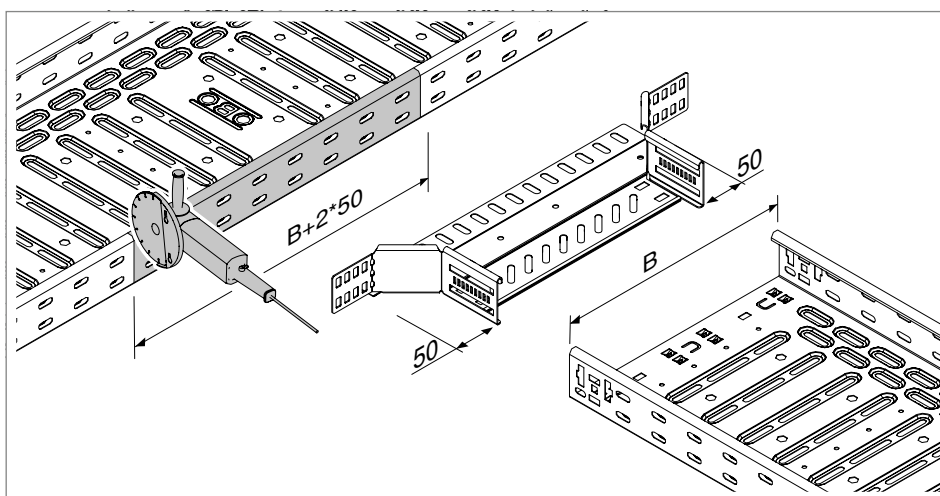
Abb. 55: Kabelrinnenholm ausklinken
