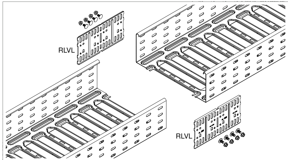
Abb. 27: Längs- und Winkelverbinder RLVL
