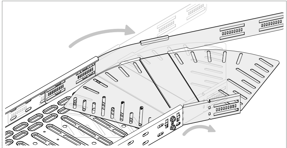
Abb. 62: Winkelverstellbaren Bogen biegen
