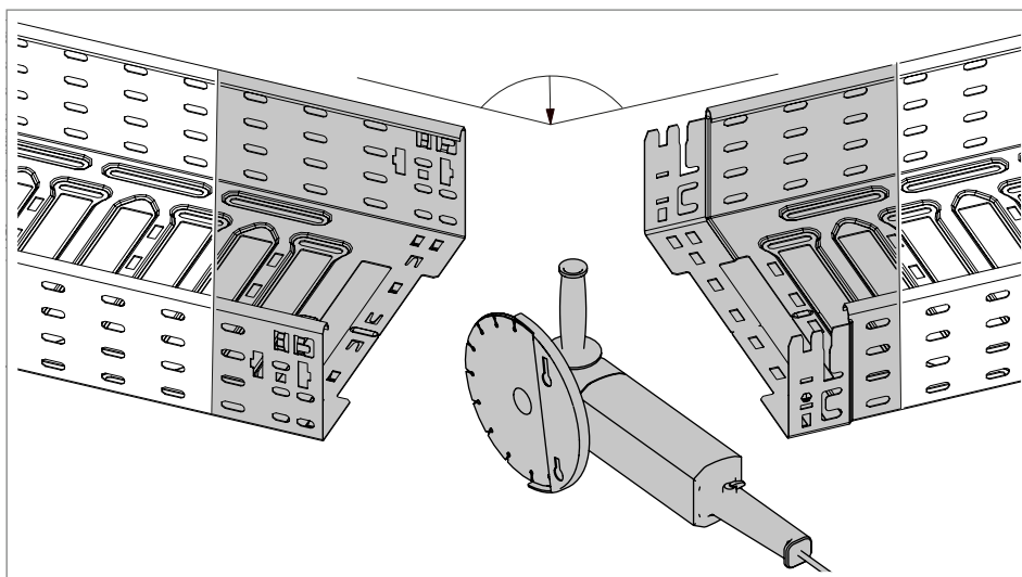
Abb. 30: Kabelrinne für Winkelerstellung schneiden
