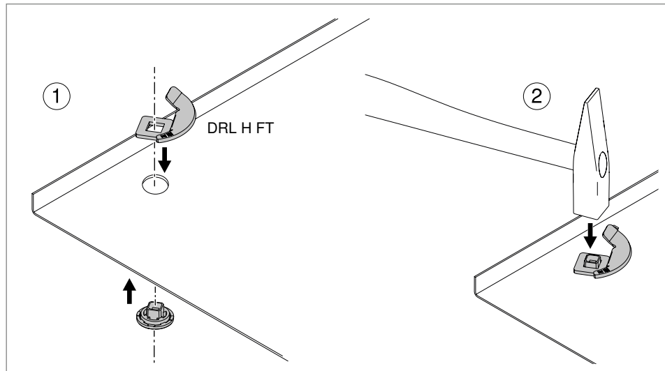
Abb. 88: Drehriegel nieten
