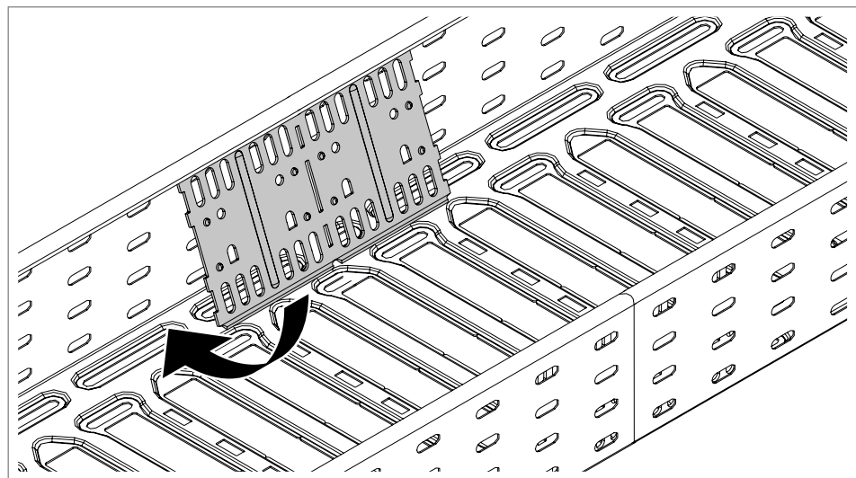
Abb. 28: Längs- und Winkelverbinder RLVL einsetzen
