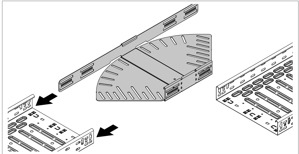
Abb. 60: Winkelverstellbaren Bogen einschieben
