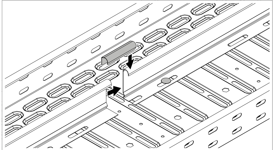
Abb. 81: Trennstege verbinden
