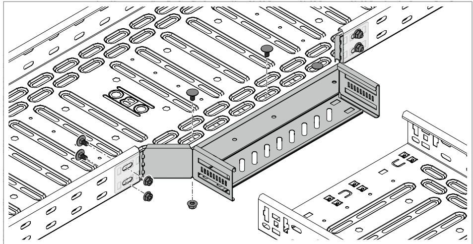
Abb. 56: Anbau-Abzweigstück an durchgehende Kabelrinne schrauben
