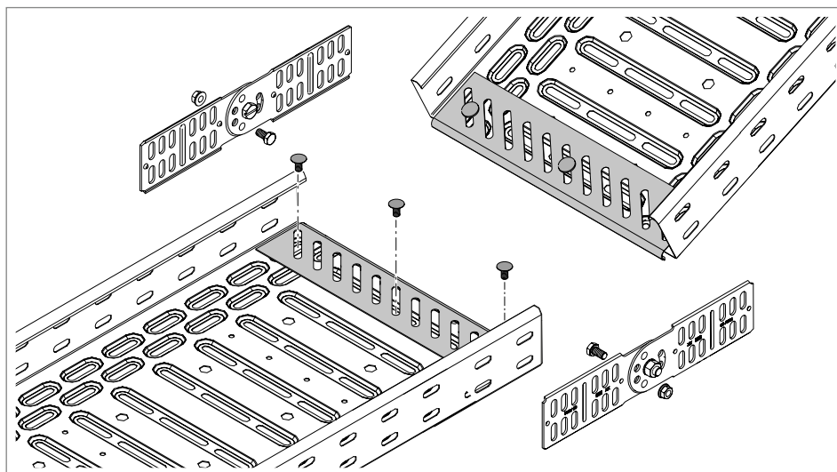
Abb. 39: Bodenendbleche anschrauben
