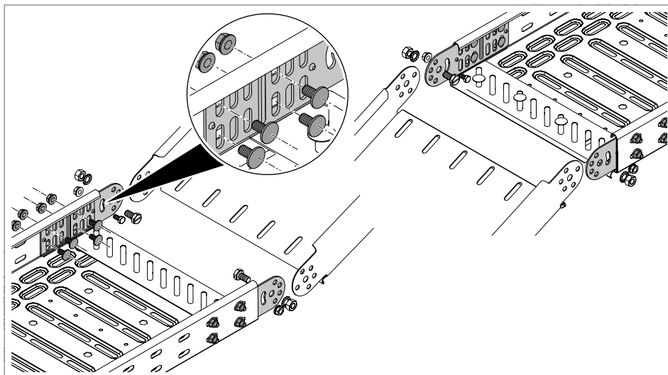
Abb. 71: Gelenkverbinder an Kabelrinnen montieren
