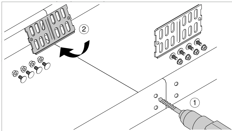
Abb. 25: Längsverbinder RLVK einsetzen
