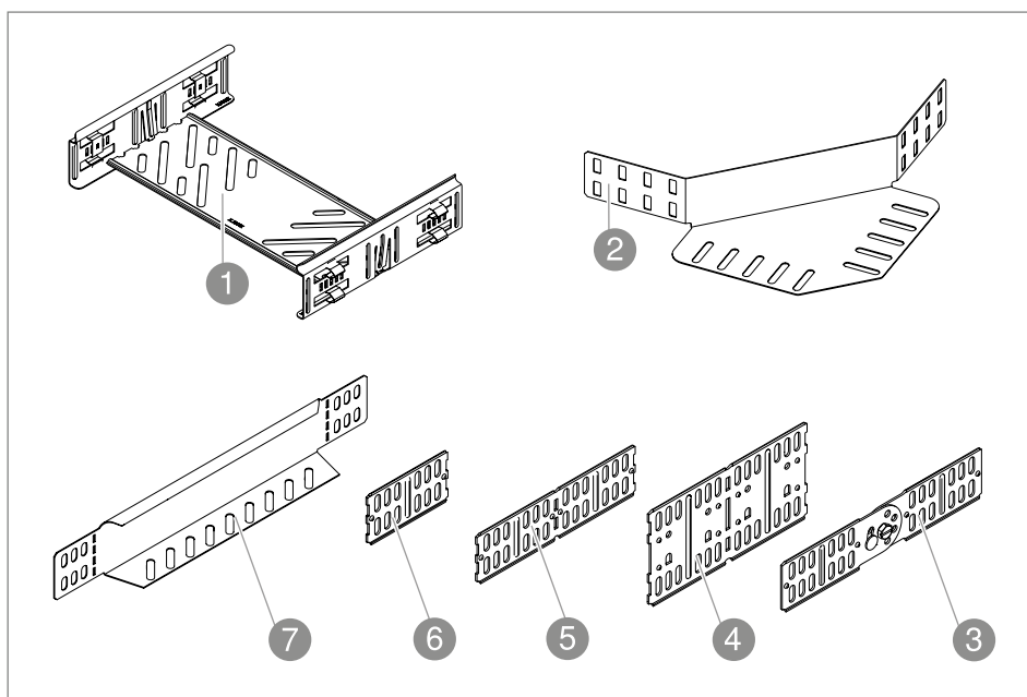
Abb. 2: Übersicht Verbinder
