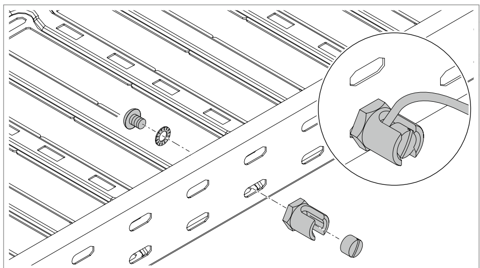
Abb. 82: Erdungsklemme montieren
