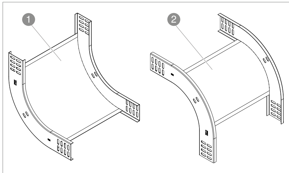
Abb. 8: Vertikalbogen steigend/fallend
