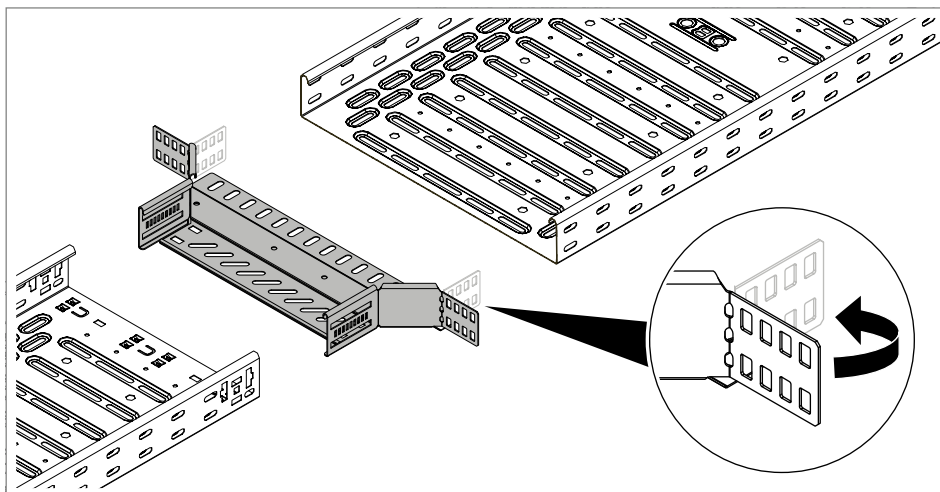
Abb. 58: Verbindungslasche biegen
