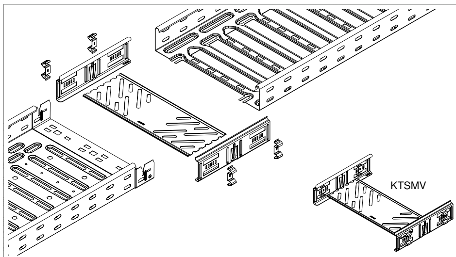
Abb. 21: Längsverbinder KTSMV
