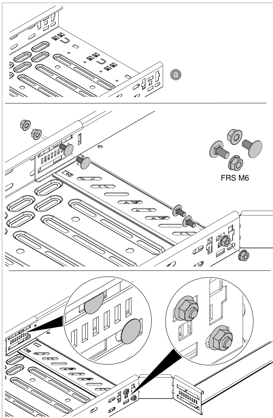
Abb. 48: Formteil mit Schrauben befestigen (Rinnenende a)
