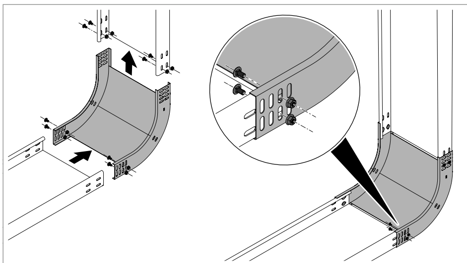
Abb. 68: Steigenden Vertikalbogen montieren
