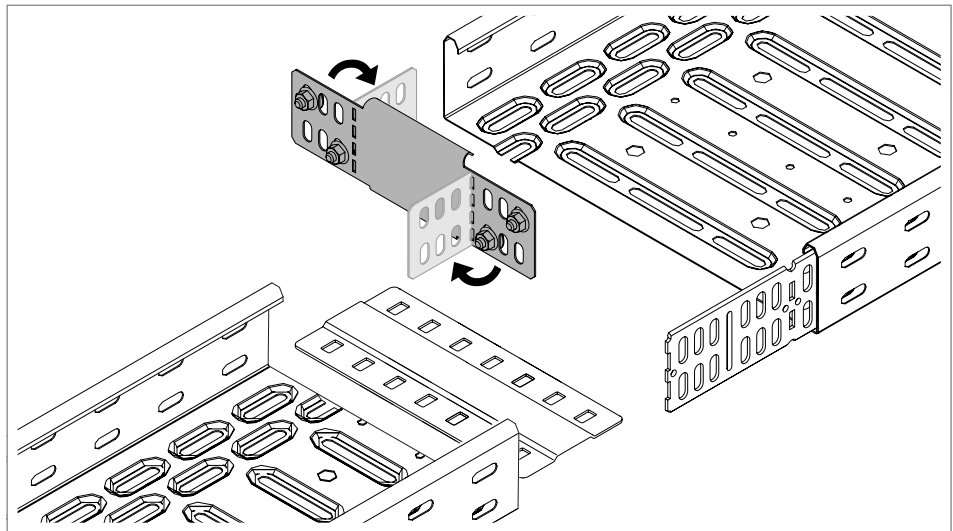
Abb. 73: Reduzierwinkel biegen
