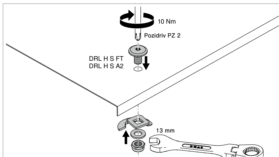
Abb. 87: Drehriegel schrauben
