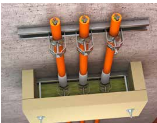
Zugentlastung Typ ZSE90-....
